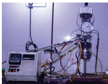
Autoclave
